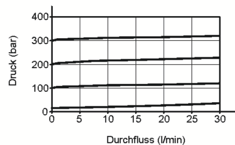
Kennlinien Einschraubventil
