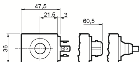
Maße Magnetspule (mm)
