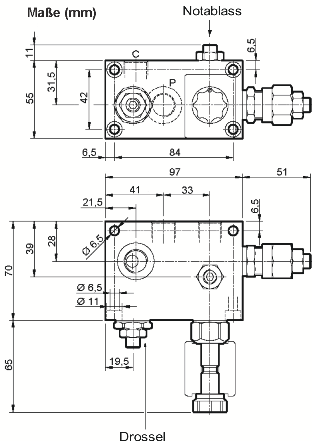
Maße Einschraubventil (mm)
