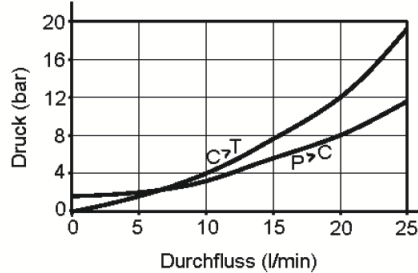
Kennlinien Hub-Senkventil
