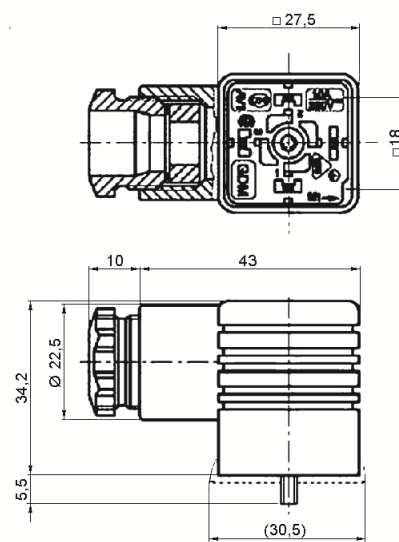
Maße Magnetstecker (mm)
