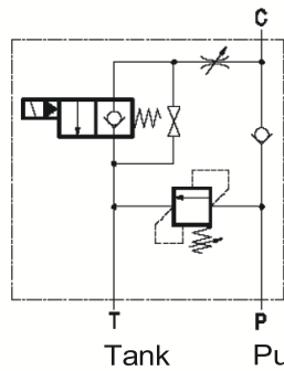
Zylinder
