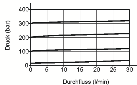
Kennlinien Einschraubventil
