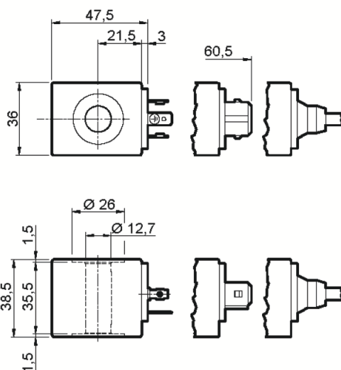
Maße Magnetspule (mm)
