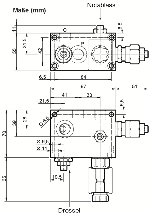
Druckbegrenzung
