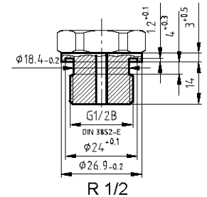
G 1/2 DIN 3852-E
